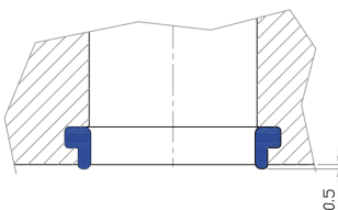
Innendichtung
