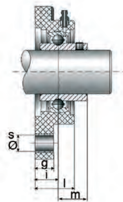
Lagereinsatz
