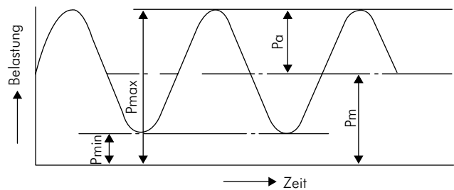
Zusammenfassung für sich wiederholende Belastungskräfte
