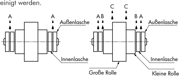
Schmierung von Kunststoffrollen
