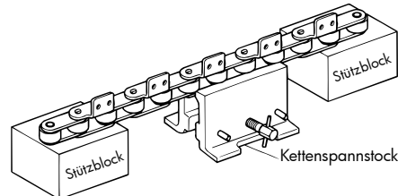
Kettenspannstock und Stützblöcke
