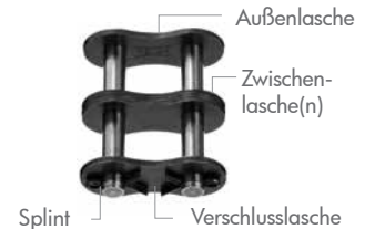
Splint Verbindungs-glied Mehrfachkette (doppelte Ausführung)
