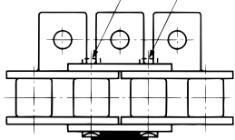
Kette mit Anbauteilen
